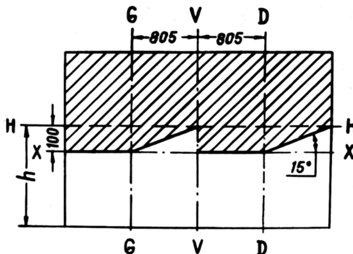
Рис. 8.2. Разметка экрана для регулировки фар: h – высота от дороги до центра фар
