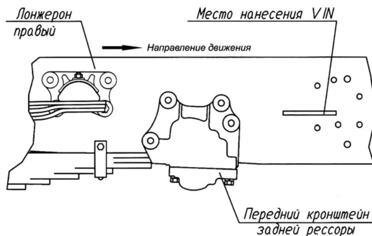
Рис. 1.1. Место нанесения VIN автомобилей и автомобильных шасси
