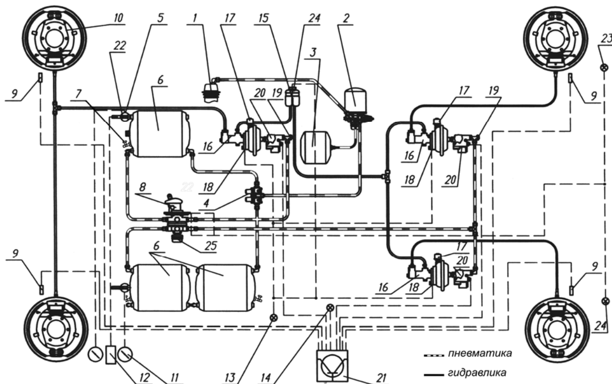
Рис. 8.3. Принципиальная схема тормозной системы автомобилей с АБС:
