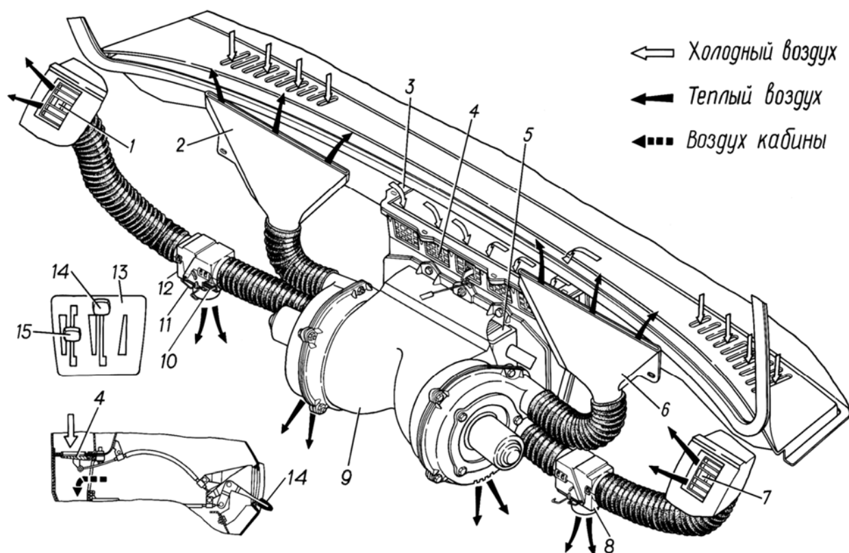
Рис. 8.1. Отопитель кабины:
