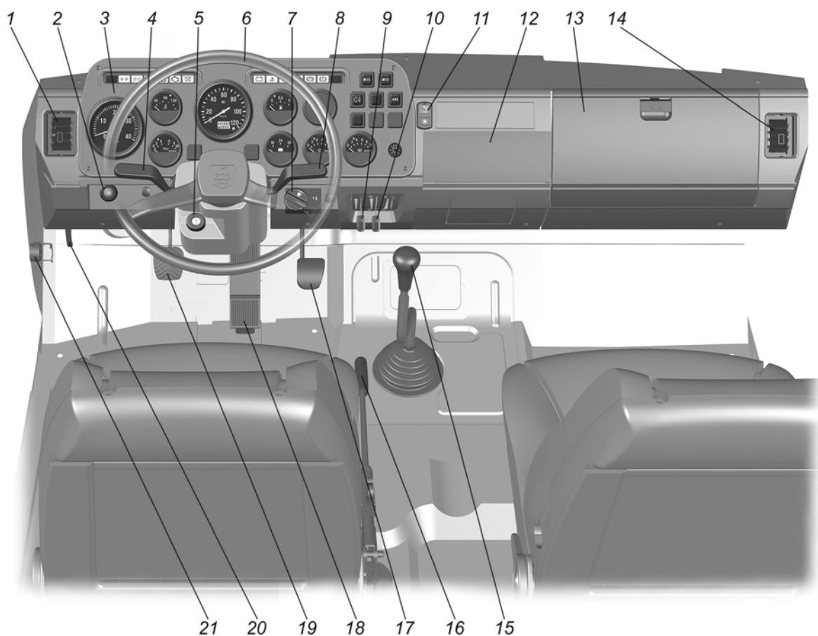
Рис. 5.1. Органы управления
