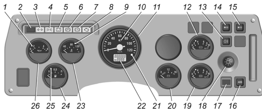
Рис. 5.13. Щиток приборов автомобиля ГАЗ-3307
