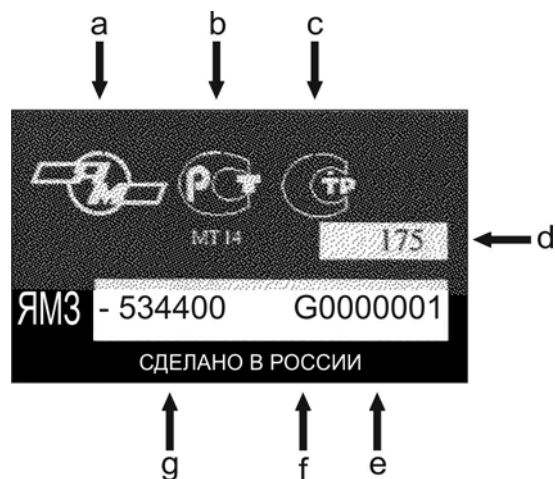
Рис. 1.4. Пример нанесение номера двигателя ЯМЗ-5344
