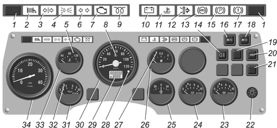
Рис. 5.10. Щиток приборов автомобиля ГАЗ-3309 с двигателем ММЗ Д-245.7 ЕЗ
