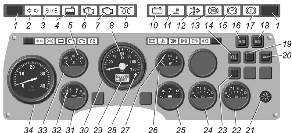
Рис. 5.12. Щиток приборов автомобиля ГАЗ-3309 с двигателем ММЗ Д-245.7 Е4 и ГАЗ-33098
